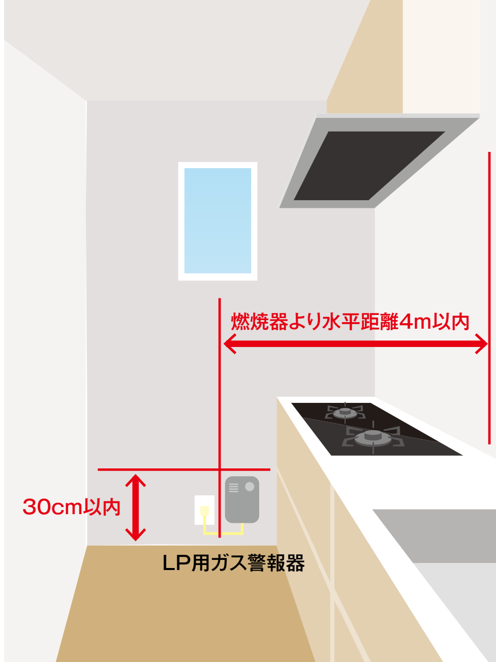
LP用ガス警報器
